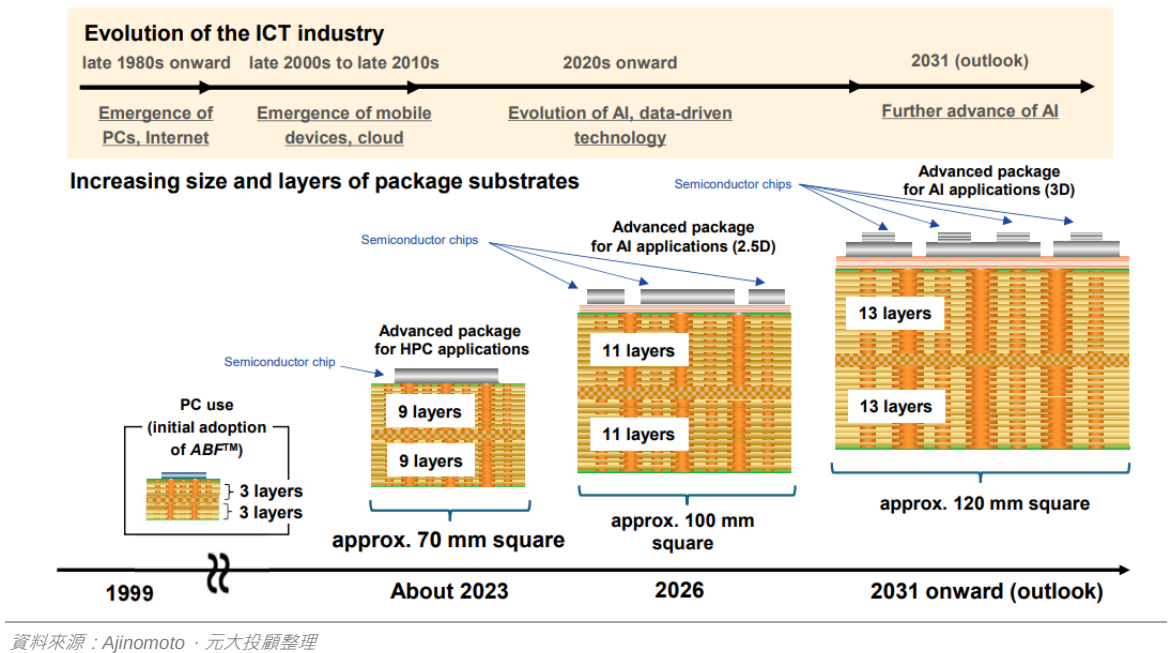
圖 3：載板面積及層數增加亦在 Ajinomoto 未來載板發展藍圖
